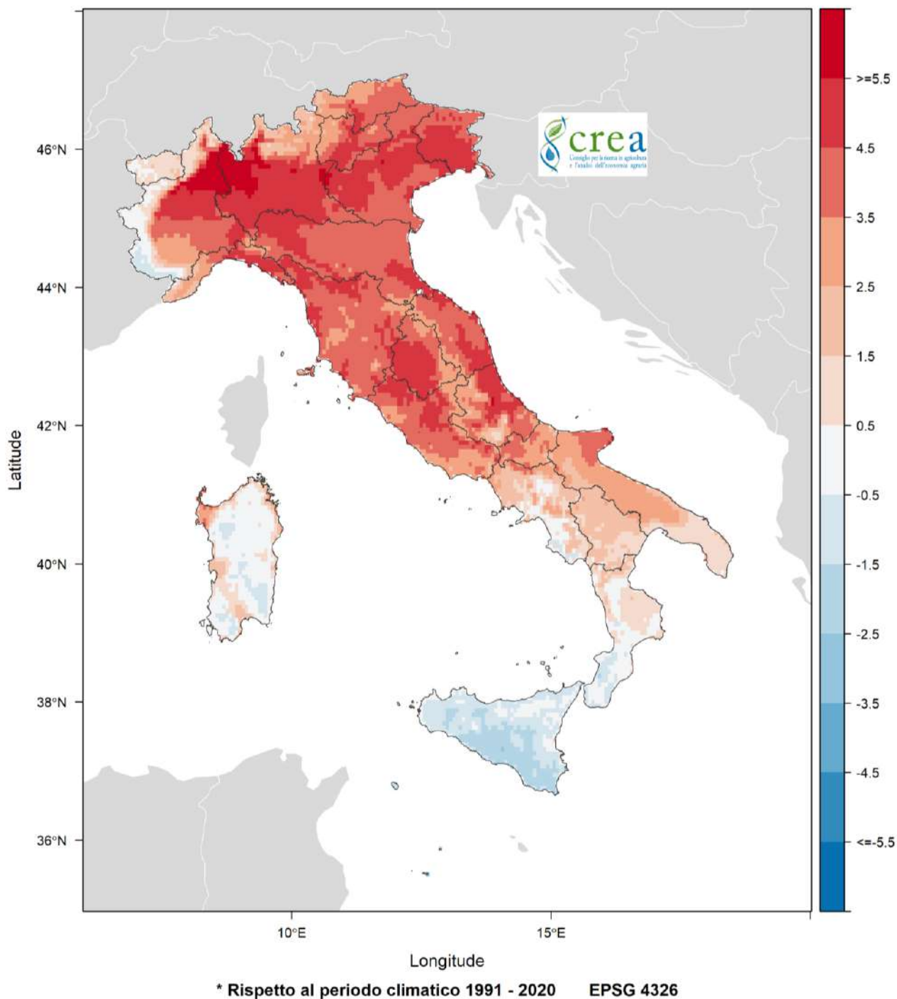
Fig. 3 - Anomalia della temperatura minima nel periodo in esame rispetto alla media 1991 - 2020. Anomaly of minimum temperature for the analyzed period with reference to the 1991-2020 mean values.
